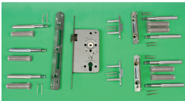
Beispiel eines (Tür-)Nachrüstsetes
